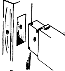
Pinned Mortise & Tenon.
