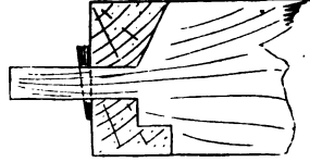
Tusk Tenon
